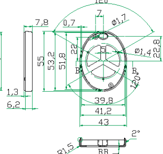
Крышка
