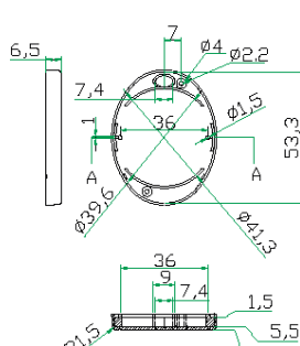
Основание
