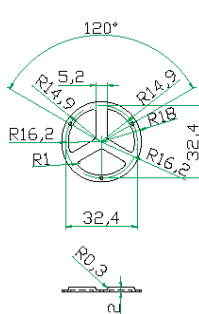
Резиновые кнопки
