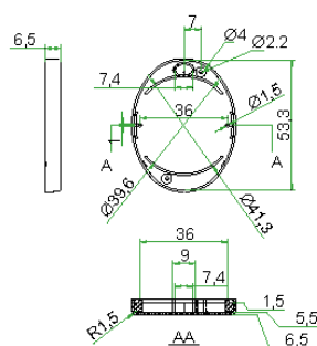
Bottom
