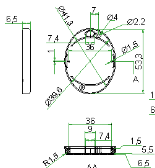
Нижняя крышка
