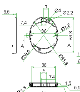
Низ корпуса
