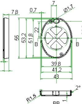
Верхняя крышка
